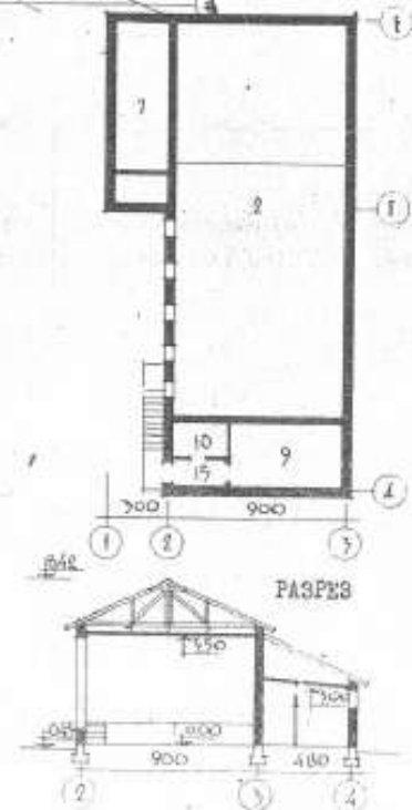
ПЛАН 2 ЭТАЖА
