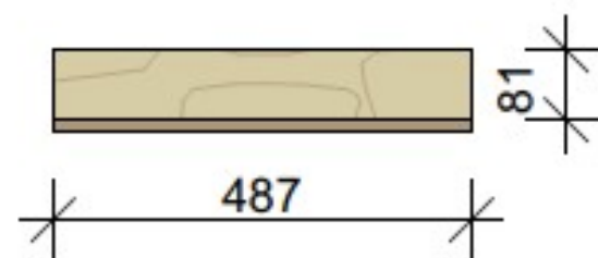
Вид сбоку, М 1:10
