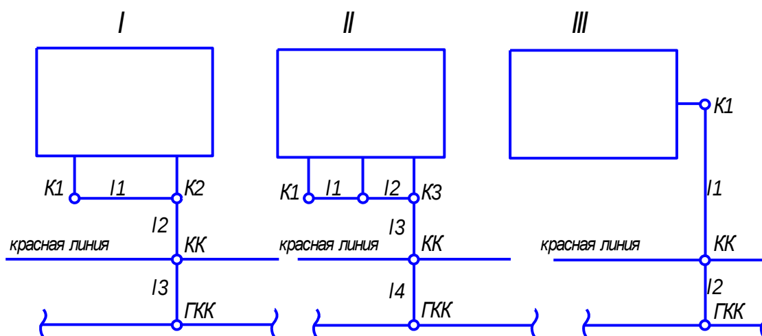
Рис.2. Уличная магистраль K1, K2, K3 - дворовые канализационные колодцы; КК - контрольный канализационный колодец; ГКК - городской канализационный колодец
