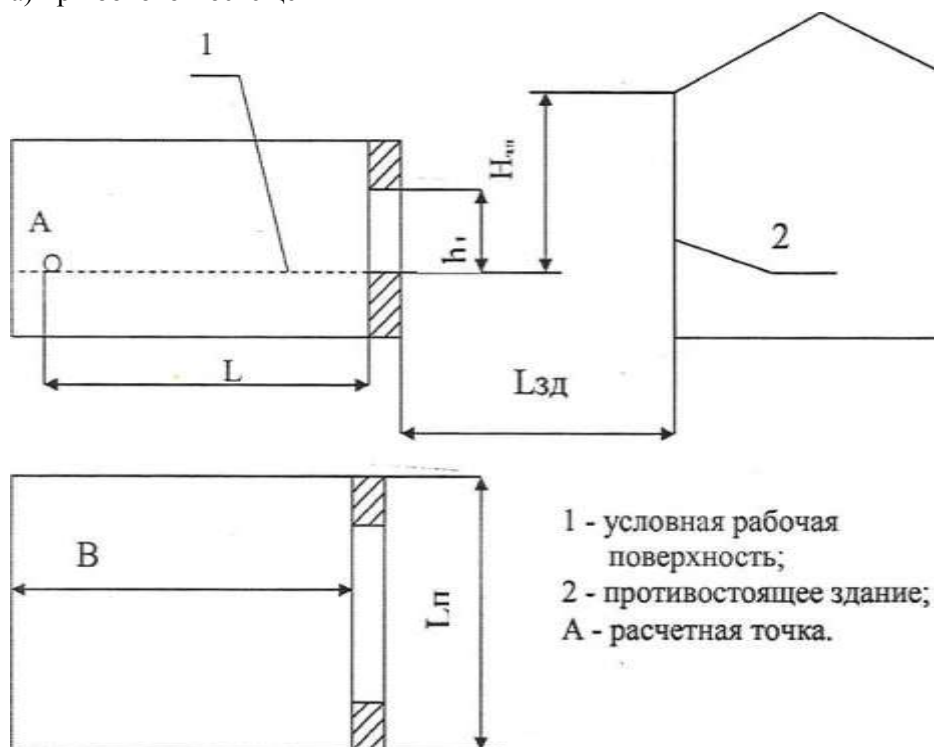
Рис. 1. Схема производственного здания
