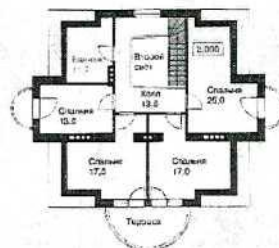
План второго этажа
