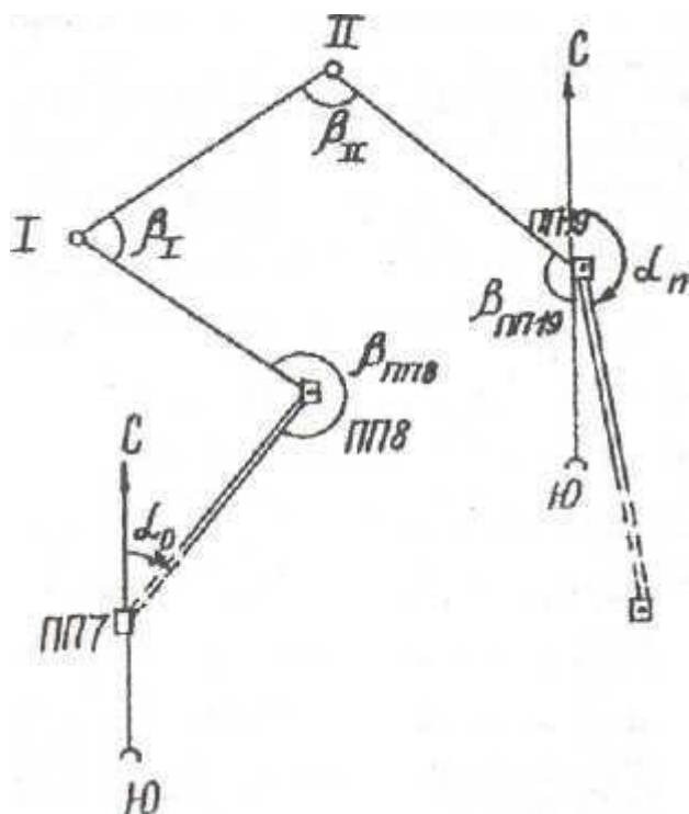
Рис. 1. Схема теодолитно-высотного хода съемочного обоснования
