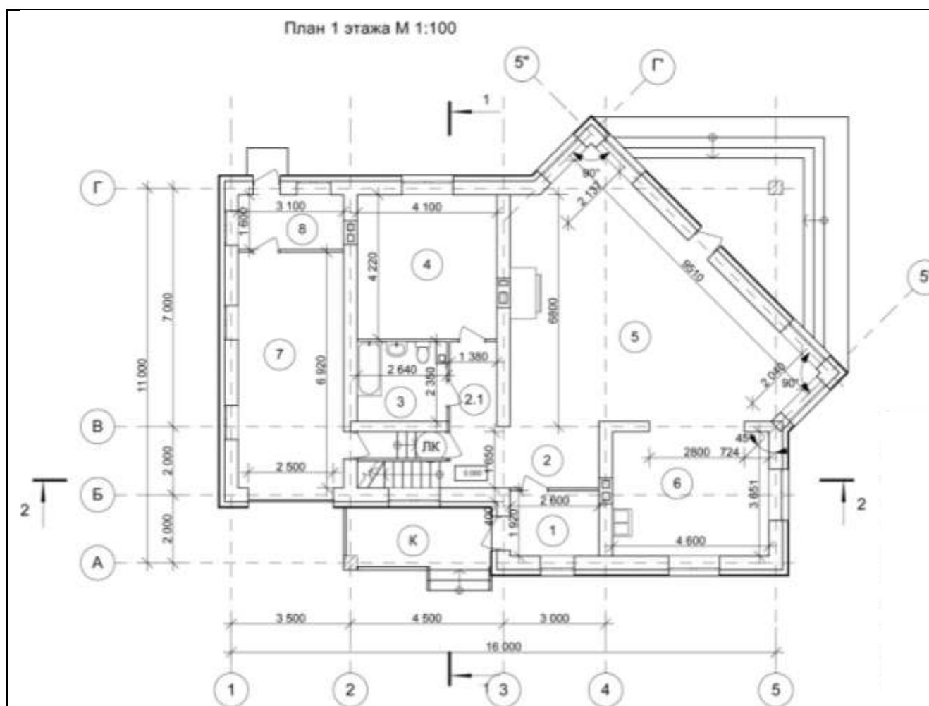
Экспликация 1 этажа
