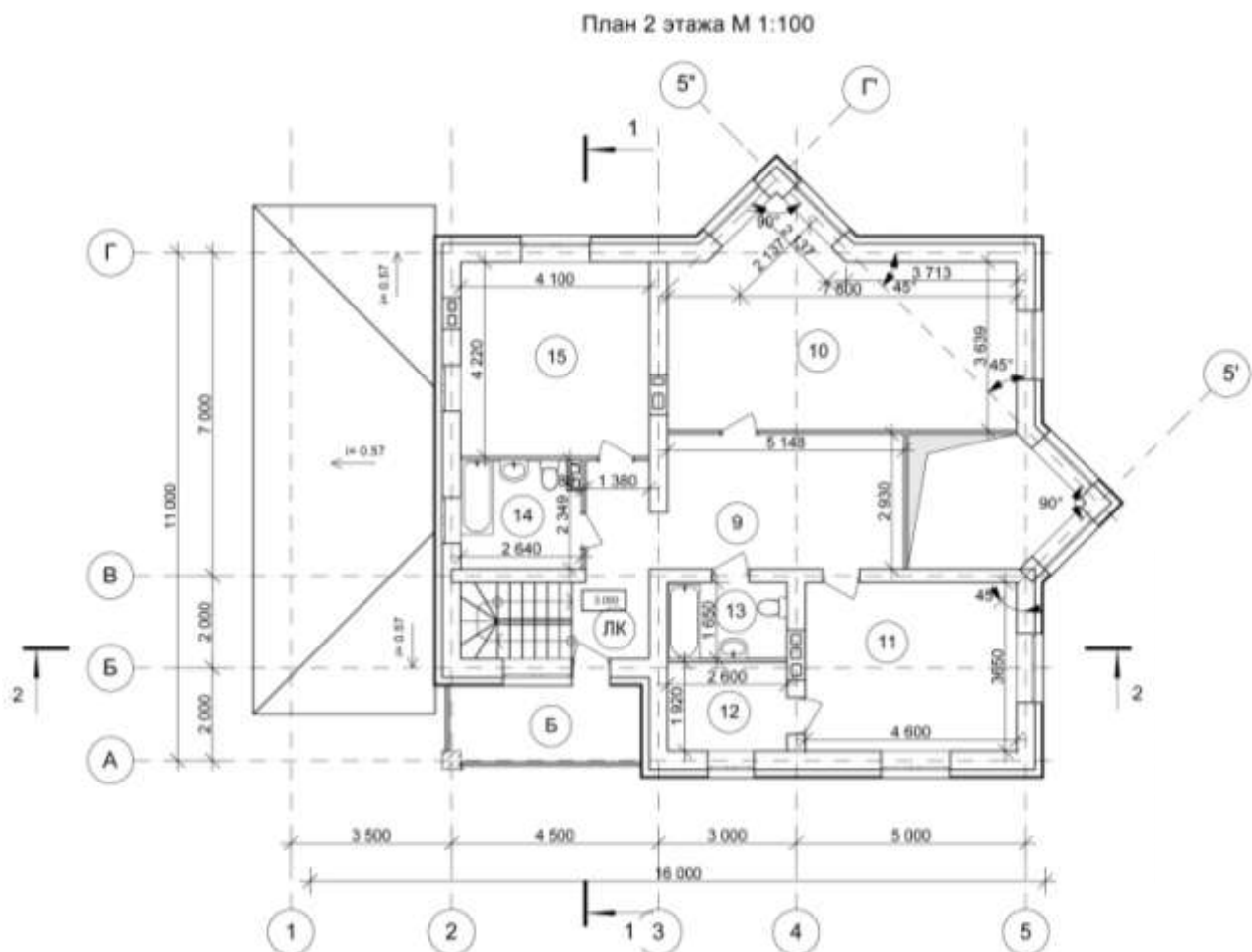
Экспликация 2 этажа
