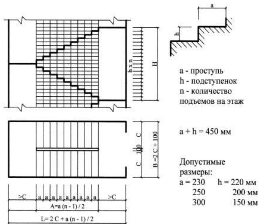
Рис. 2. К расчету лестничной клетки
