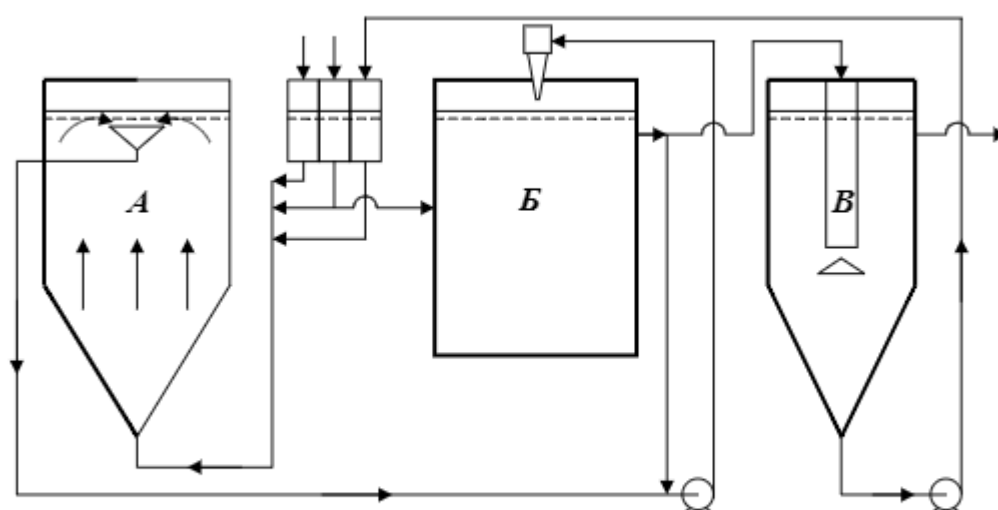
Схема нитри-денитрификатора
