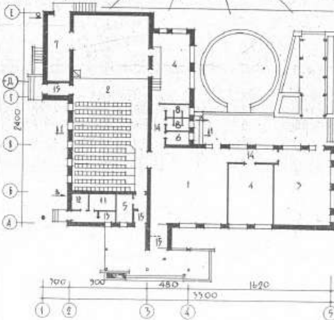
ПЛАН 1 ЭТАЖА
