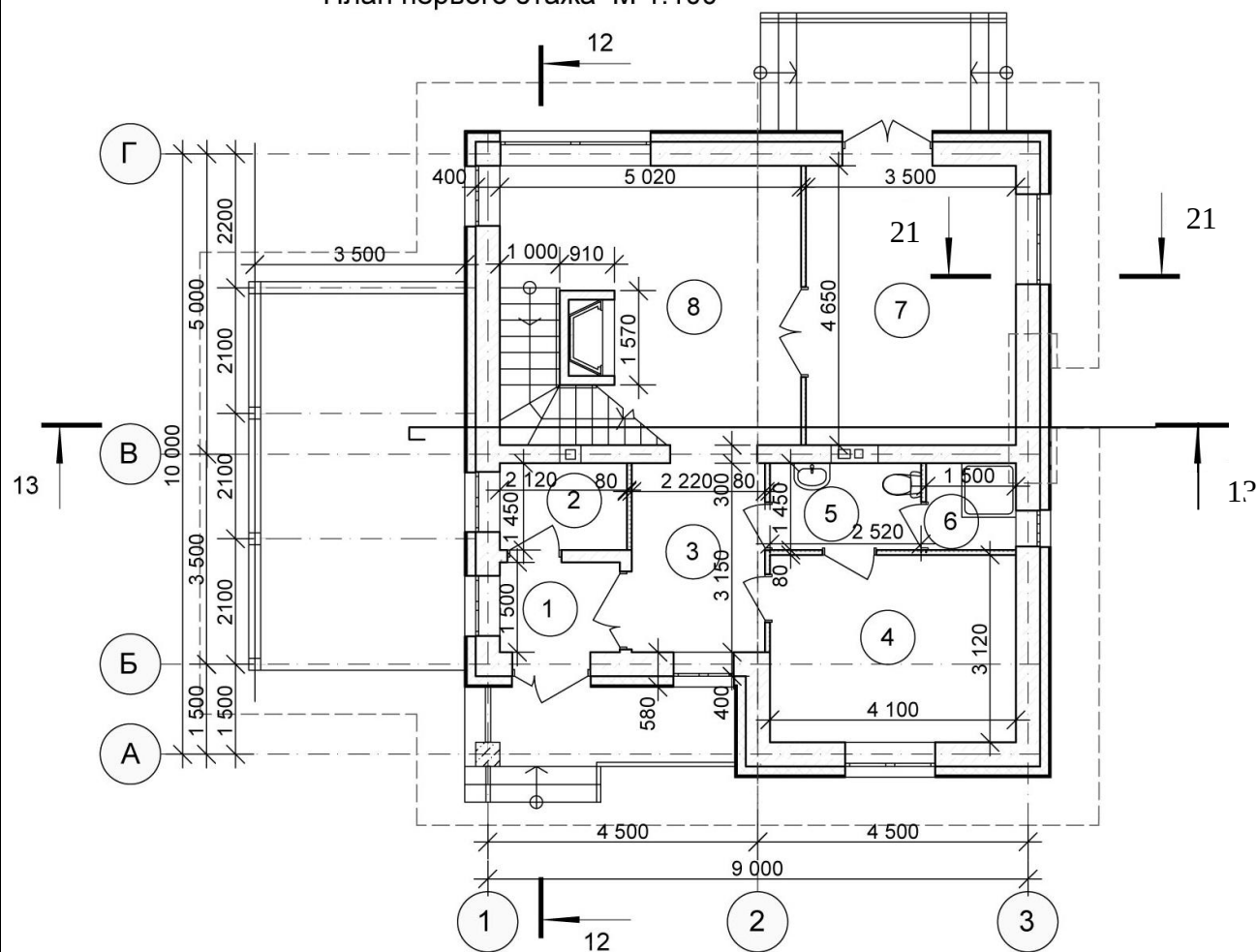
Экспликация помещений
