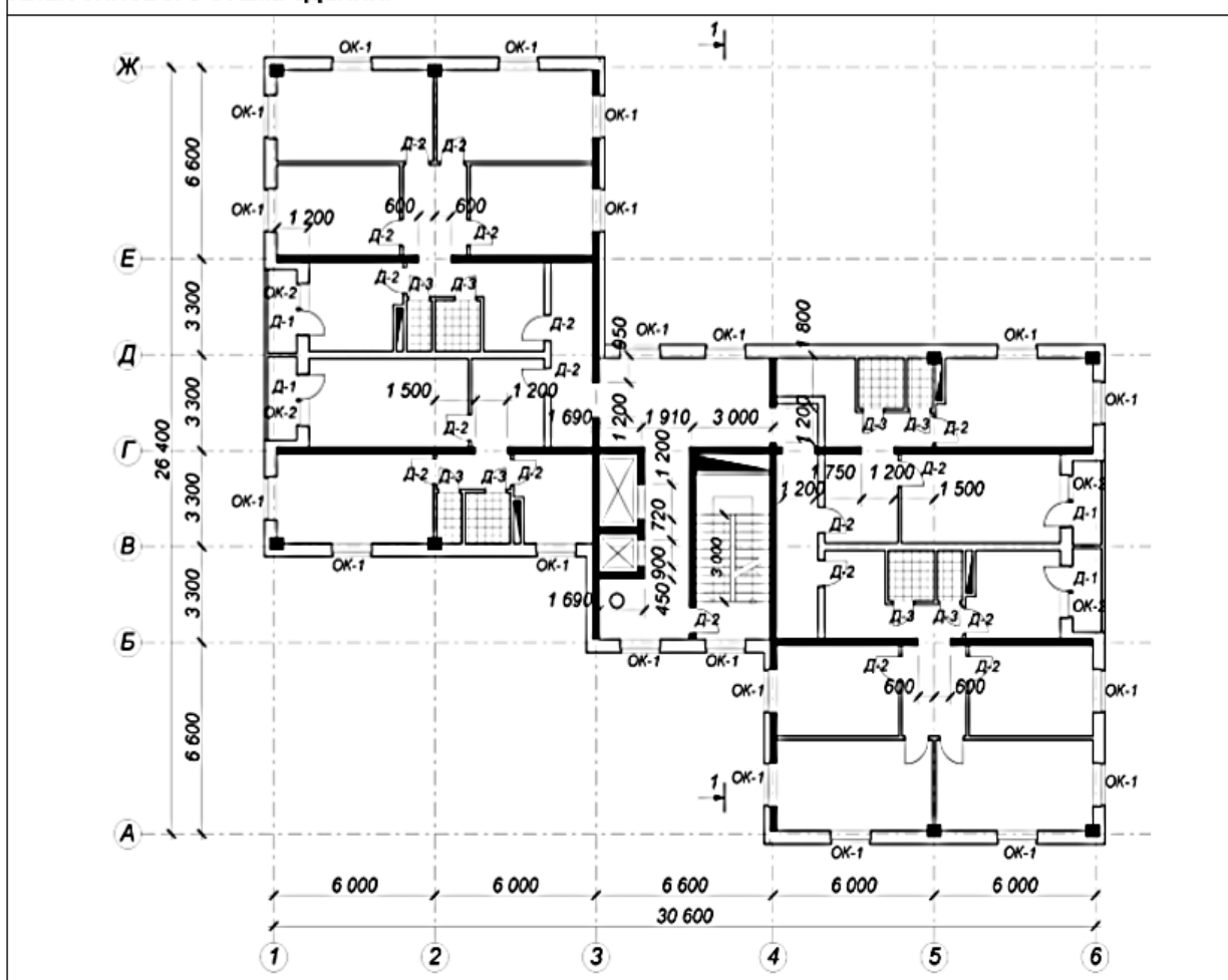
План типового этажа здания:
