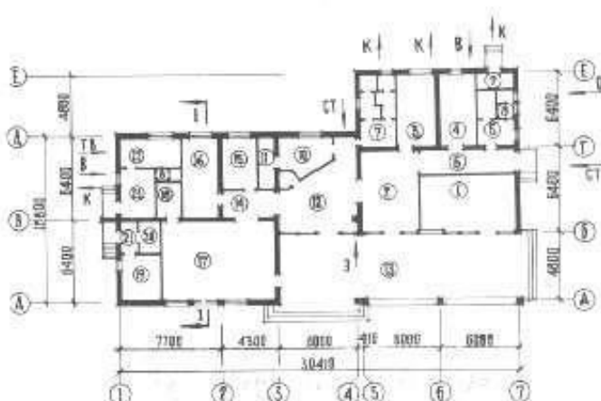
ПЛАН ЭТАЖА
