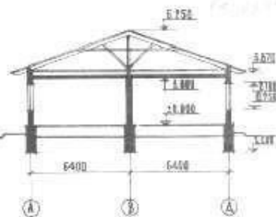
РАЗРЕЗ I-I
