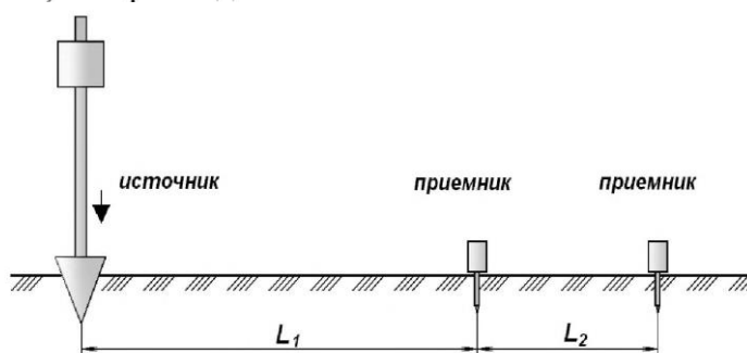
Рис.1.11. Измерение поперечных волн
