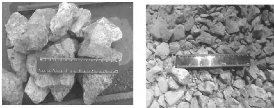
Рис. 3.7. Исходный материал и продукт дробления экспериментального образца виброщековой дробилки
