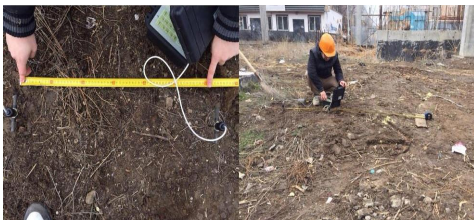
Рис.1.13. Получение продольной волны на глинистом грунте
