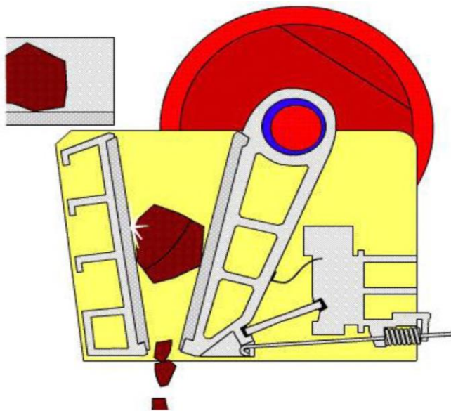
Рис.2.2.Щековая дробилка с простым движением щеки
