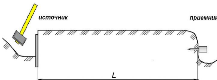
Рис.1.11. Измерение поперечных волн
