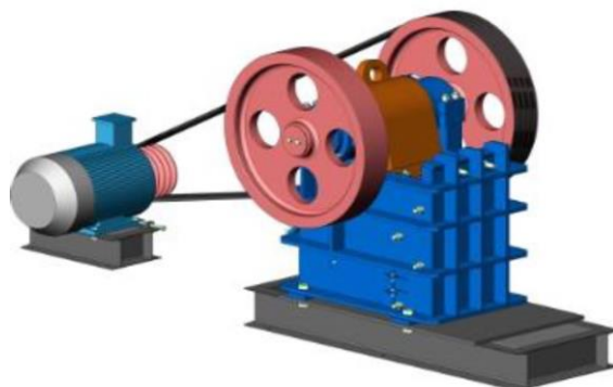
Рис.2.3. Щековая дробилка со сложным движением щеки
