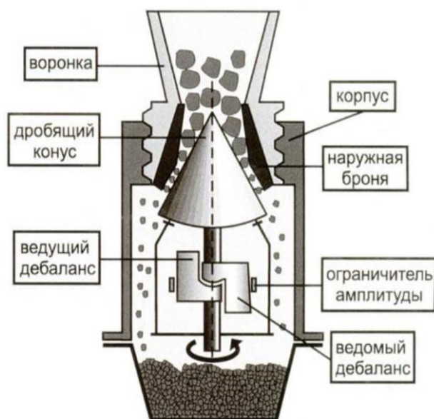
Рис. 2.4. Конусная дробилка с крутым дробящим конусом
