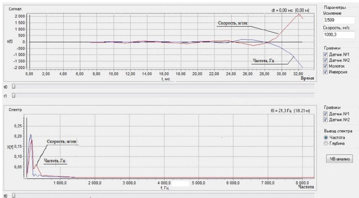
Рис.1.15. График зависимости частоты от скорости полученной продольной волны
