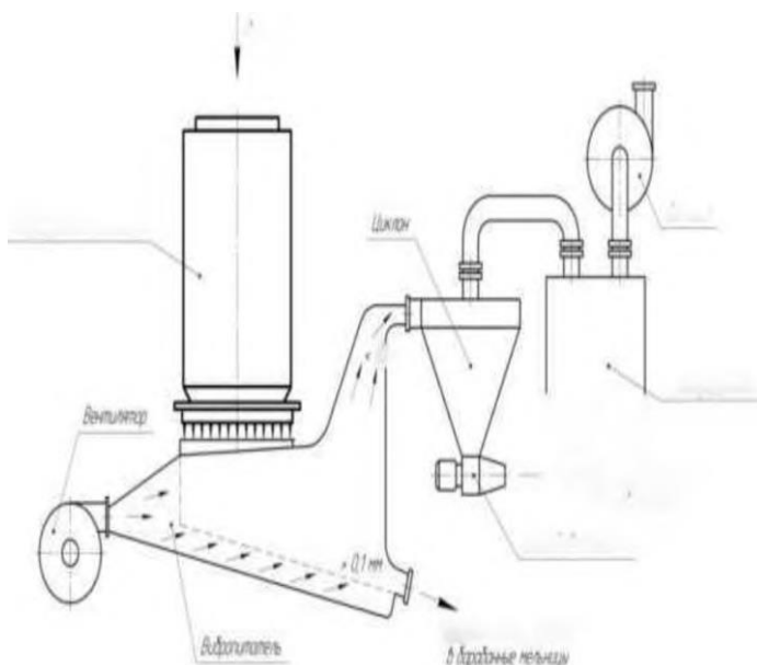
Рис. 3.11. Схема модернизации участка помола клинкера
