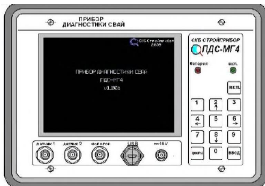
Рис. 1.3. Лицевая панель электронного блока ПДС-МГ4
