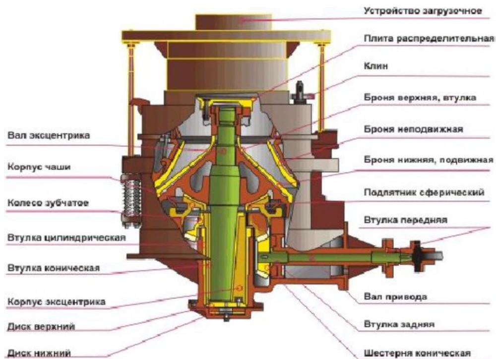
Рис. 2.6. Валковая дробилка
