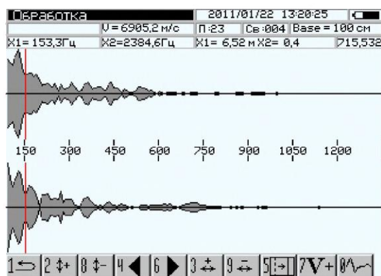
Рис 1.10. Спектр сигнала
