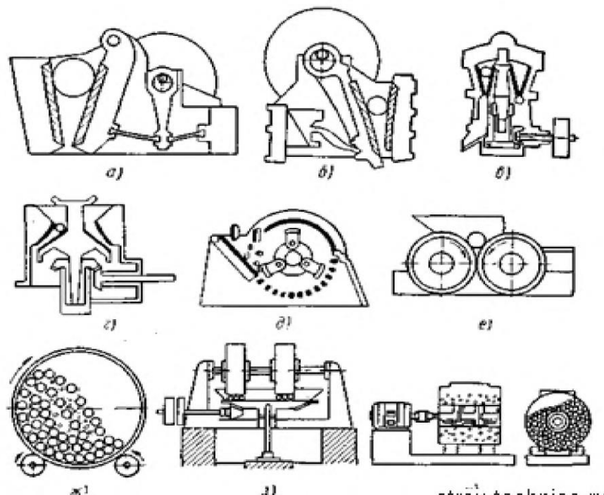
Рис.2.1. Схемы дробильных машин:
