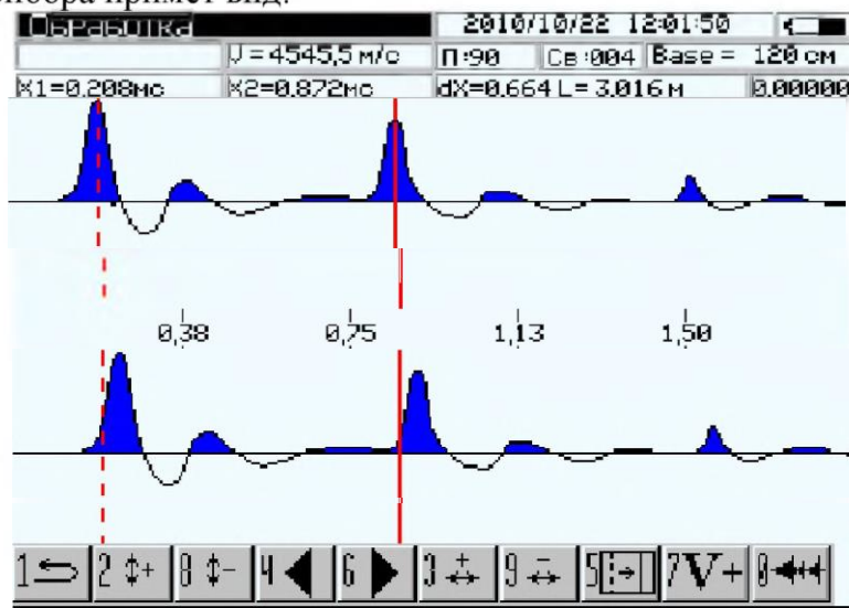
Рис 1.9. Индикатор записи сигнала
