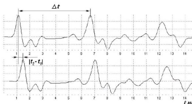
Рис. 1.2. Измерение начальным воздействием и отраженной волной
