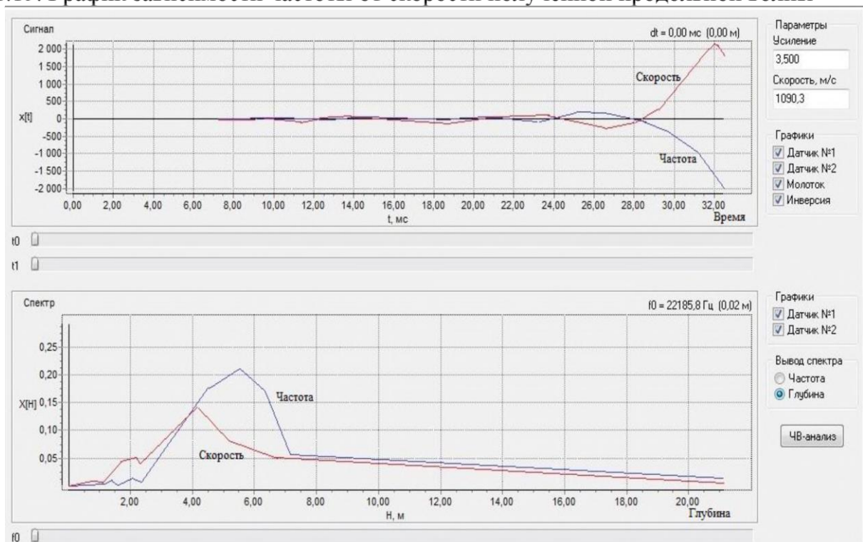
Рис.1.16. График зависимости частоты от скорости полученной продольной волны
