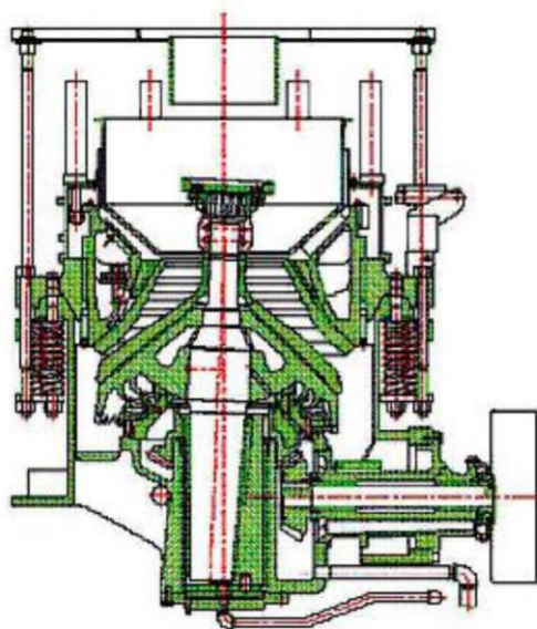
Рис. 2.5. Конусная дробилка с пологим дробящим конусом
