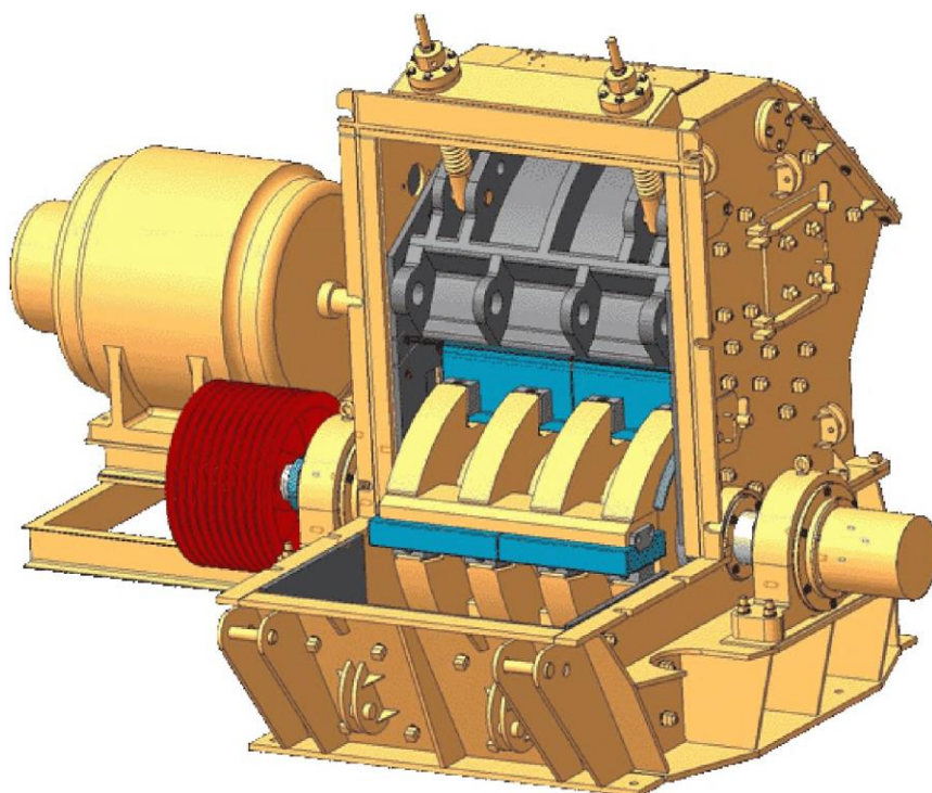
Рис. 2.8. Роторная дробилка.
