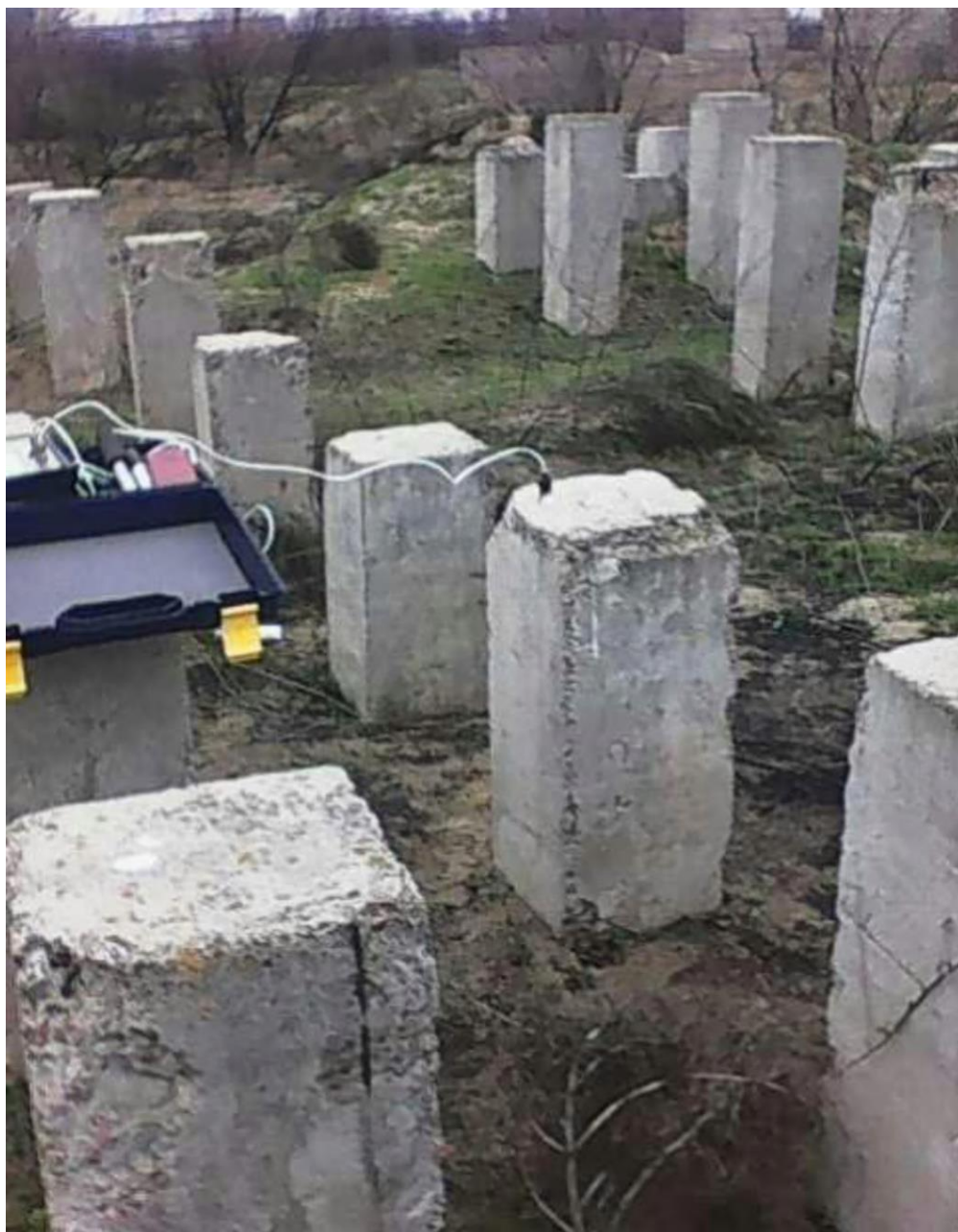
Рис. 1.19 Испытание свайного поля
