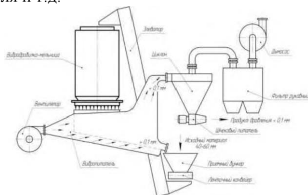
Рис. 3.10. Схема установки для «сухого» помола
