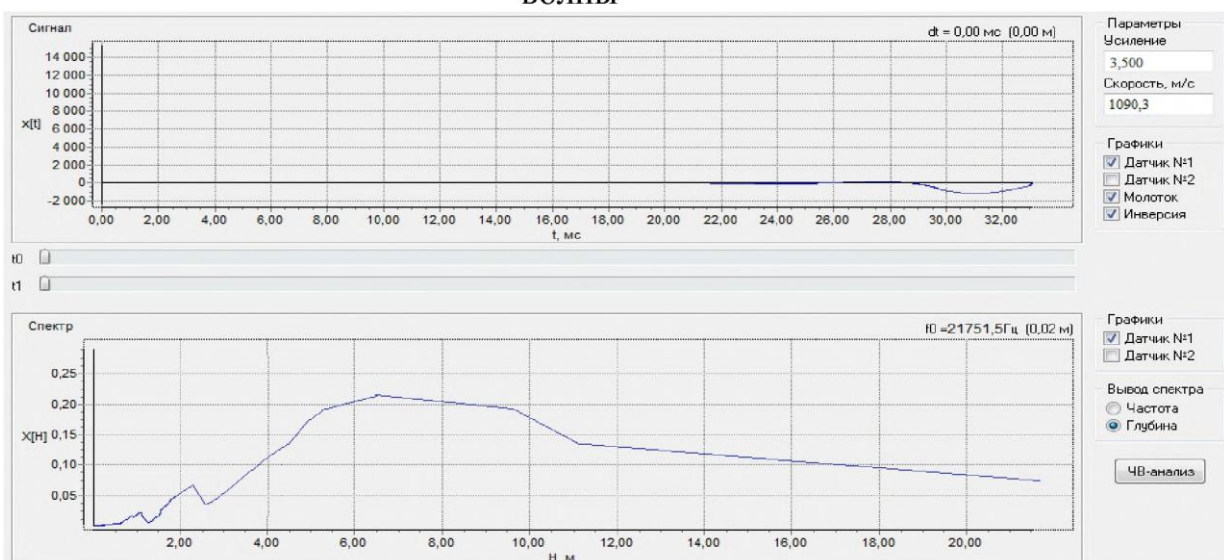
Рис.1.18. График зависимости частоты от скорости полученной продольной ВОЛНЫ
