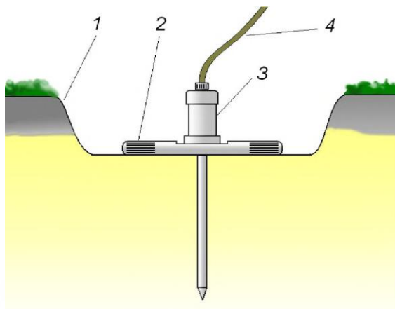
Рис. 1.8. Крепление сейсмоприемника на грунте 1 – верхний слой грунта; 2 – приспособление для крепления сейсмоприемника на грунт; 3 – сейсмоприемник; 4 – кабель сейсмоприемника
