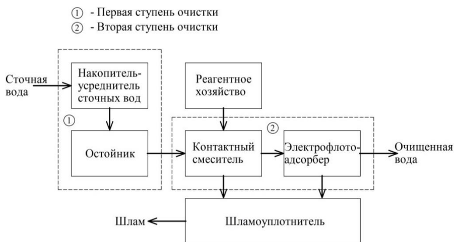
Рис. 2. Технологическая блок-схема поэтапной очистки СВ, образующихся на ТФ
